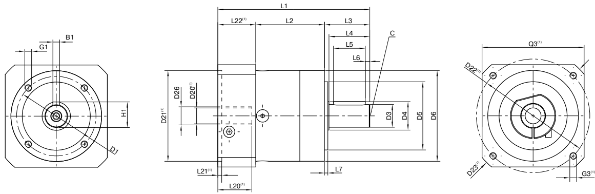
Darstellung entspricht einem PLE060 / 1-stufig / Abtriebswelle mit Passfeder / 11 mm Spannsystem / Motoranpassung – einteilig / B5 Flanschtyp Motor Drawing corresponds to a PLE060 / 1-stage / output shaft with feather key / 11 mm clamping system / motor adaptation – one part / B5 flange type motor
